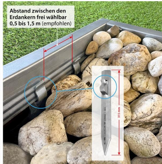
Befestigung mit Erdanker GEA604315
